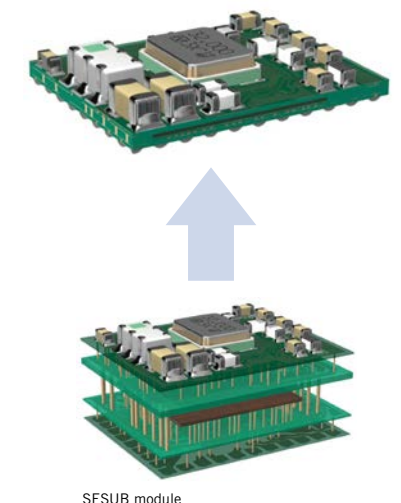
SESUB module
